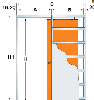
Tokborítás elemei
