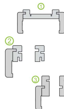
Tokborítás elemei
